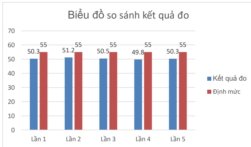
Hình 4. Kết quả đo của máy quạt sử dụng 4 cánh quạt
