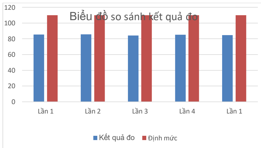
Hình 5. Kết quả đo của máy lạnh hoạt động mức thấp nhất
