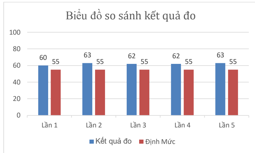
Hình 3. Kết quả đo của máy quạt sử dụng 5 cánh quạt
